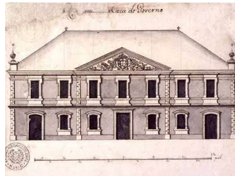
3. Projeto para a Casa de Governo de Santa Catarina
