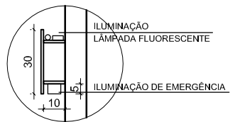
DETALHE CAIXA PASSAGEM ENERGIA 2o. PAVTO.
